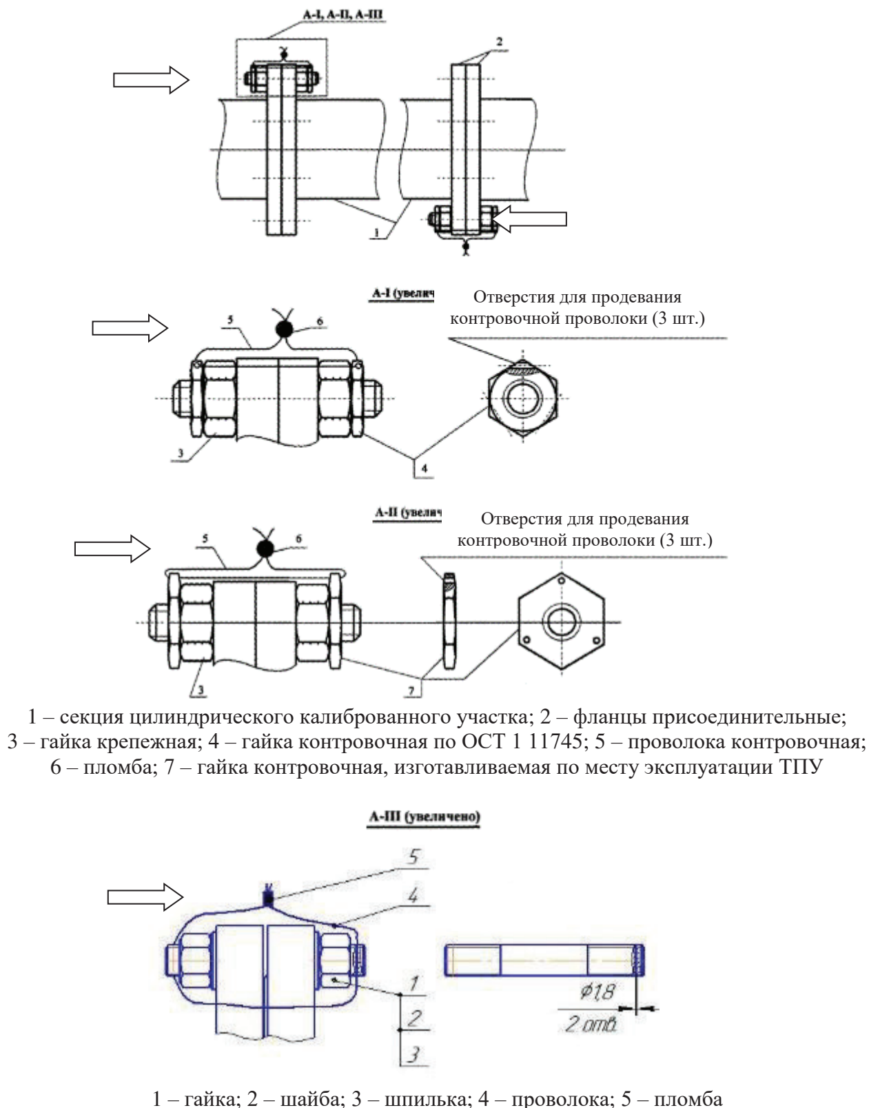
Рисунок 2 – Схема пломбирования от несанкционированного доступа, обозначение места нанесения знаков поверки на фланцевые соединения калиброванного участка ТПУ
