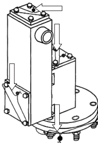
Рисунок 3 – Схема пломбирования от несанкционированного доступа, обозначение места нанесения знаков поверки на детекторы ТПУ
